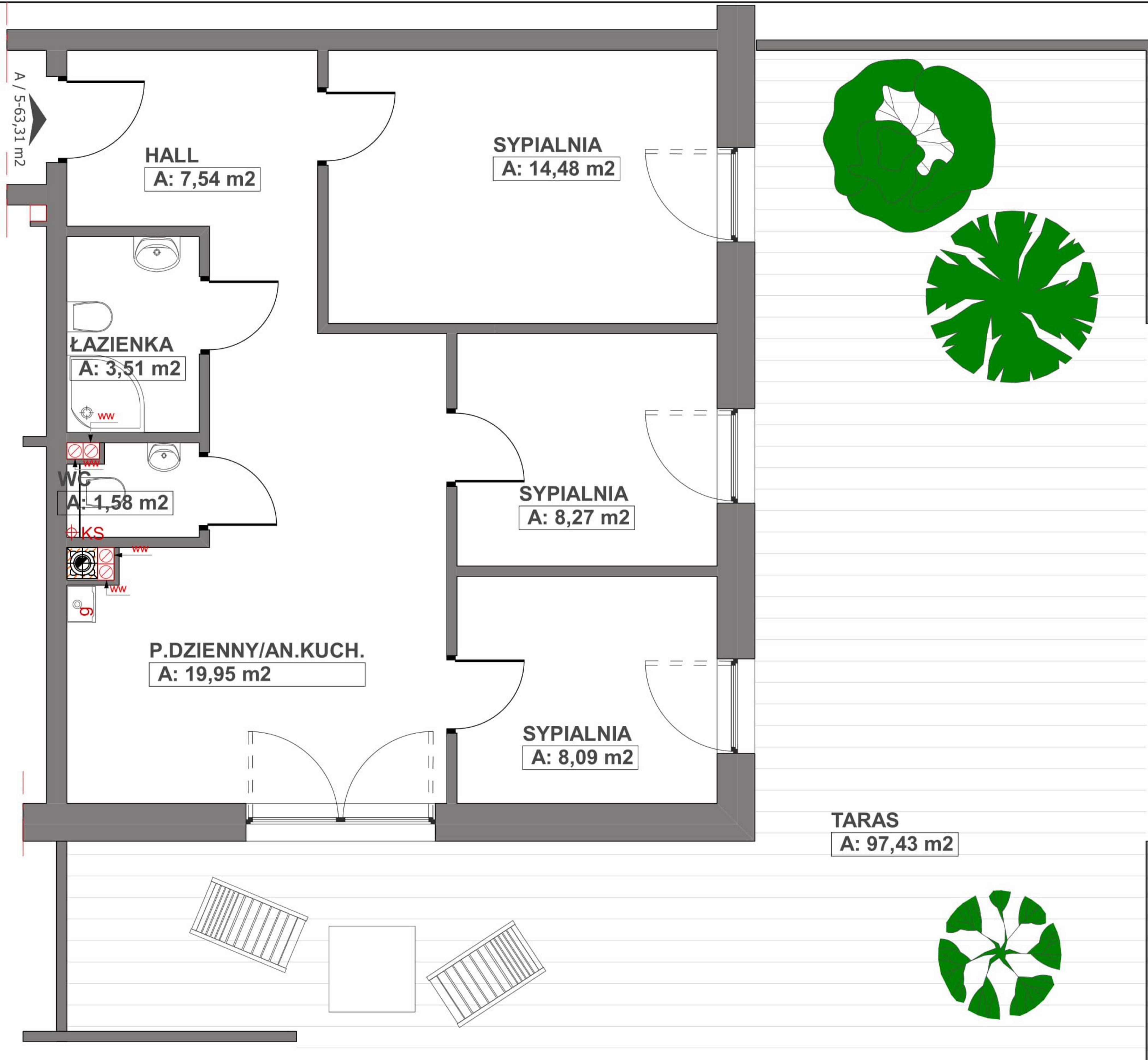
BUDYNEK A-PARTER- A5 - 63,31 m 2
